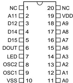
HT6187 - 20 SOP
