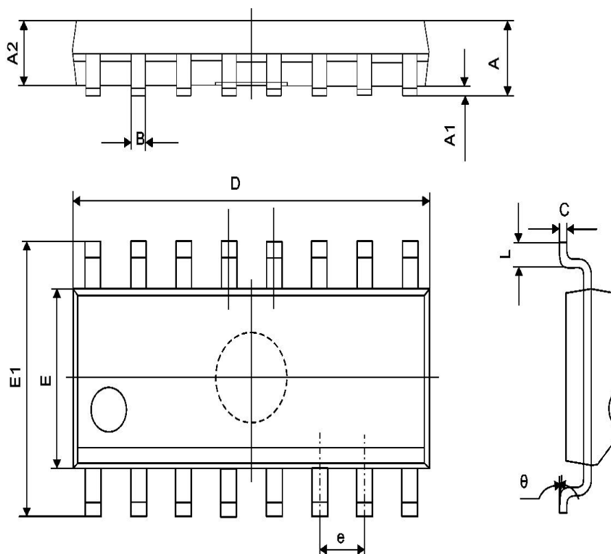
CKE8102M SOP16 封装图
