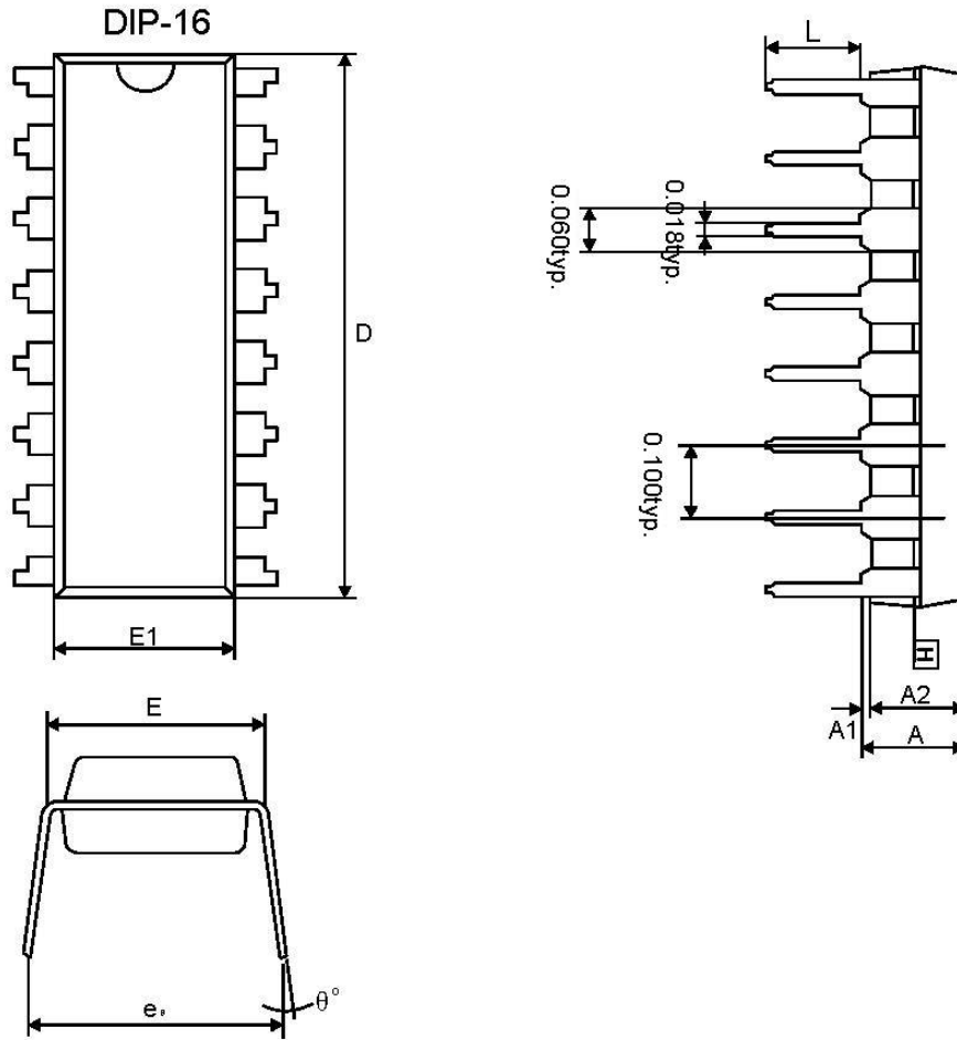
CKE8102M DIP16 封装图
