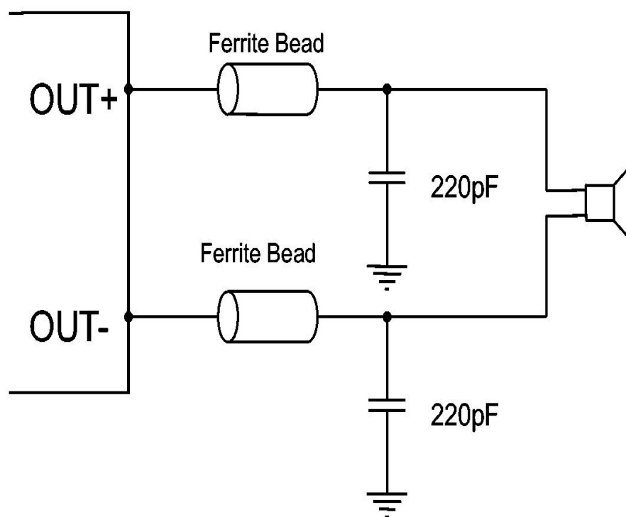
使用磁珠滤波器减小 EMI
