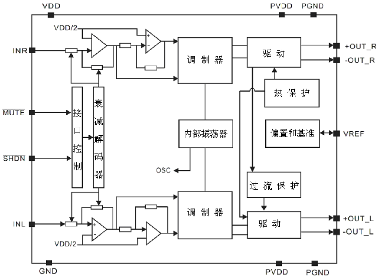
CKE8102M 原理框图
