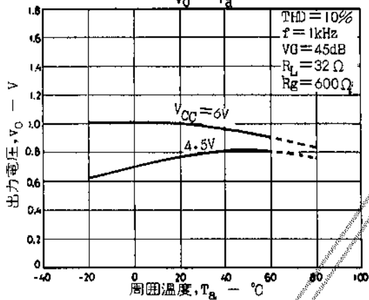
パワーアンプ v_o - T_a
